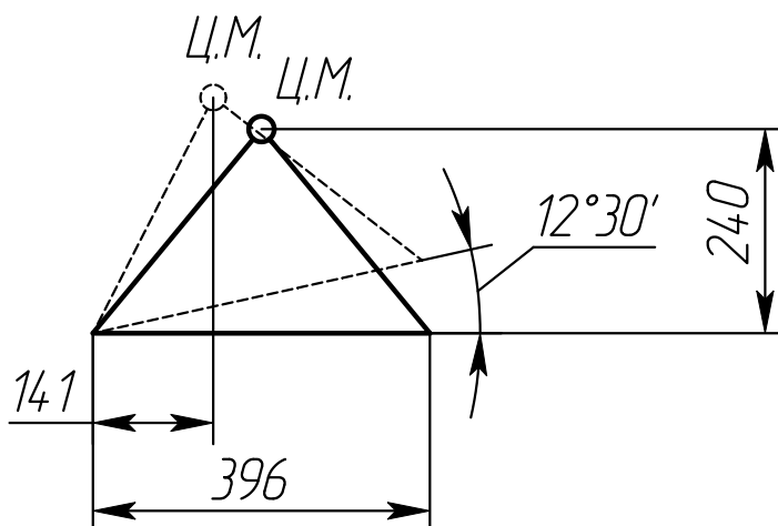
Рисунок 1- Схема устойчивости электронасосного агрегата типа ВС32
